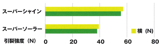
既存製品(スーパーソーラー)との強度比較
